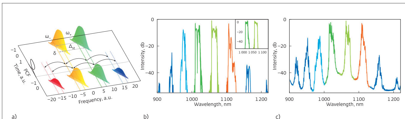
Рис. 1. Генерация спектрального комба чирпованных импульсов: а) нелинейное смешение в фотонно-кристаллическом световоде двух коротких импульсов с линейной частотной модуляцией, \Delta\omega – разница частот между импульсами, \delta – расстояние между продольными модами внутри импульсов; (b-c) спектр сигнала на выходе нелинейного световода в расчете (b) и эксперименте (c)
